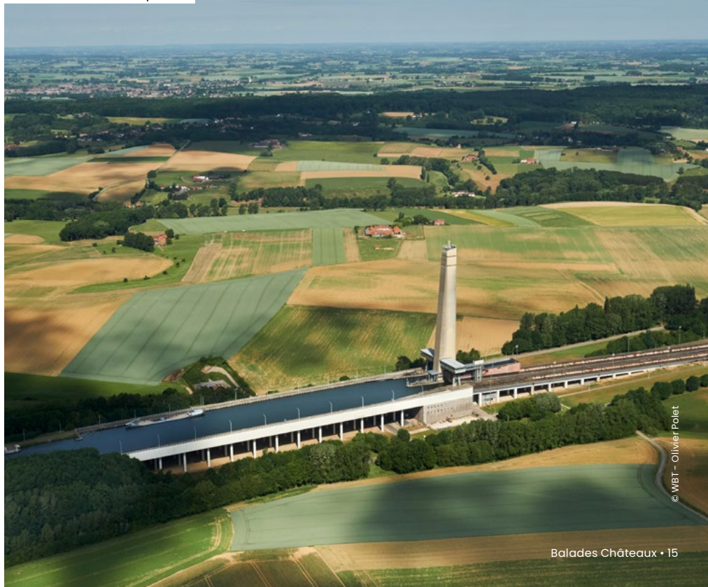
Plan incliné de Ronquières
